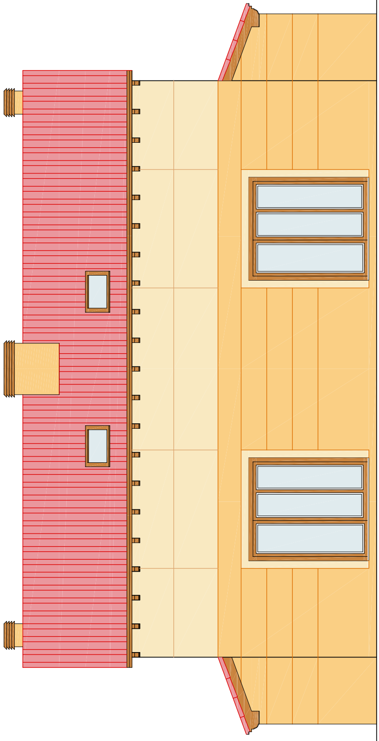
ALZADO SUROESTE
