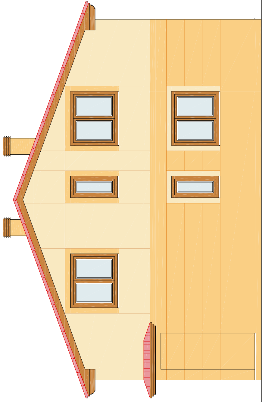
ALZADO SURESTE
