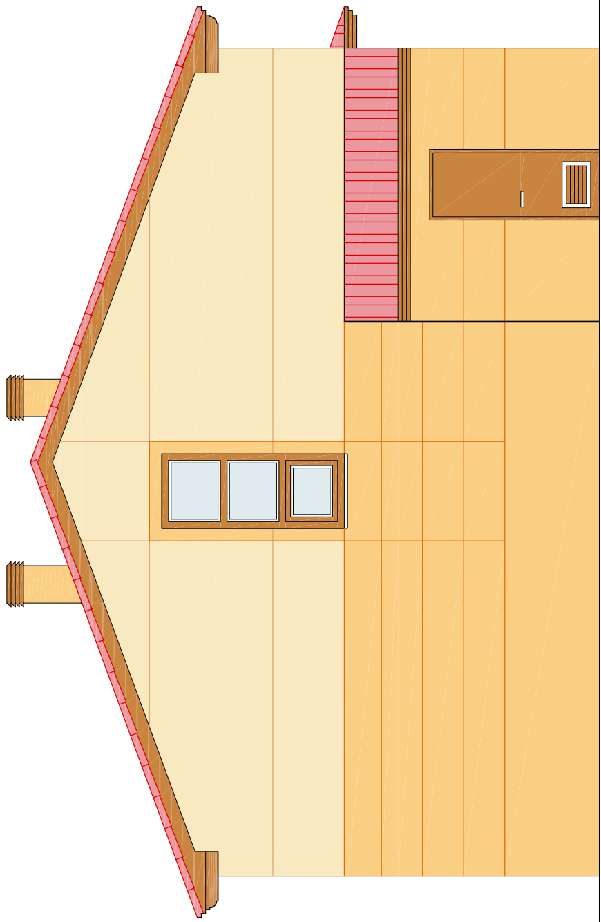
ALZADO NOROESTE
